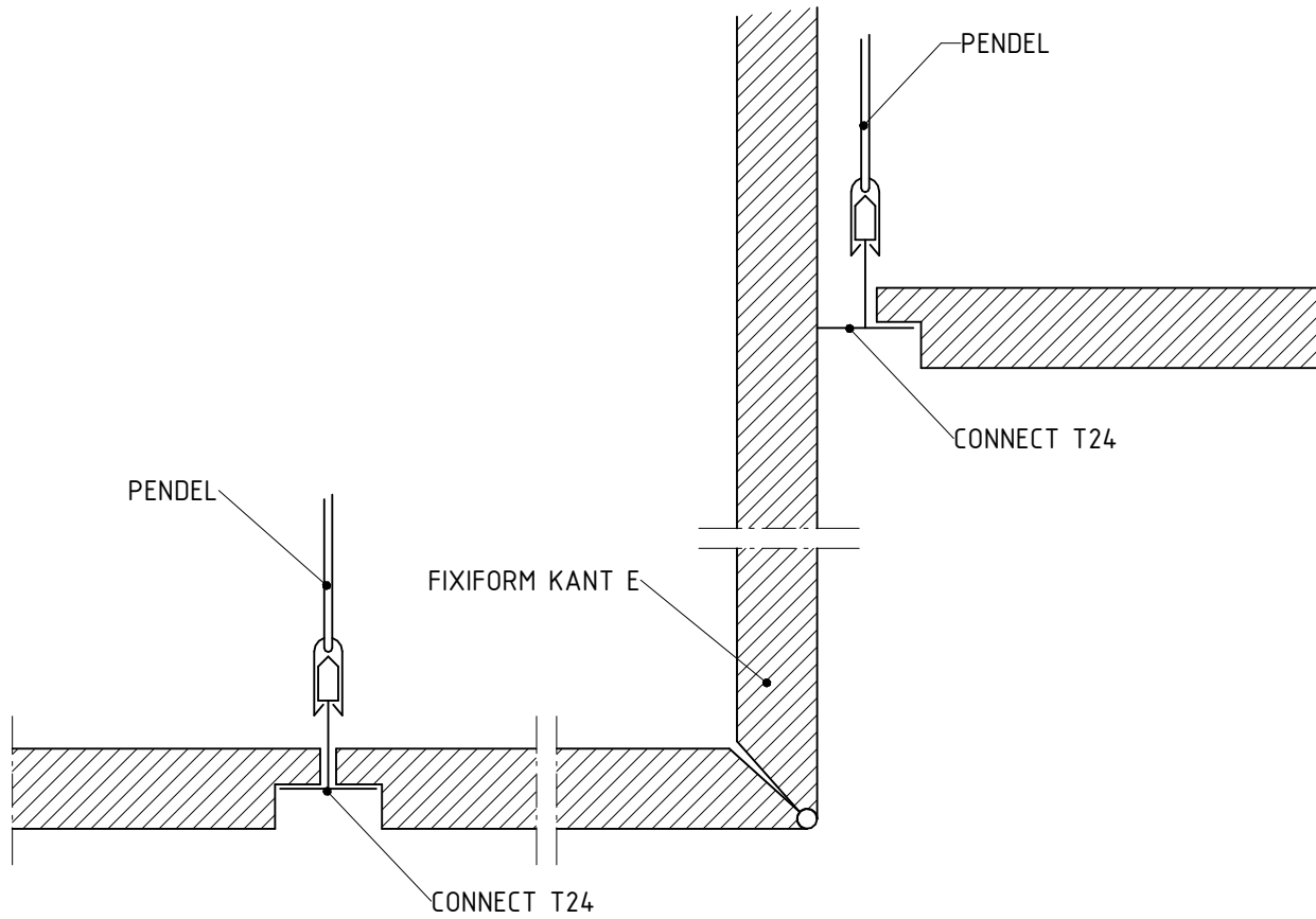
UTD05 - NIVÅSKILLNAD 1 : 2
