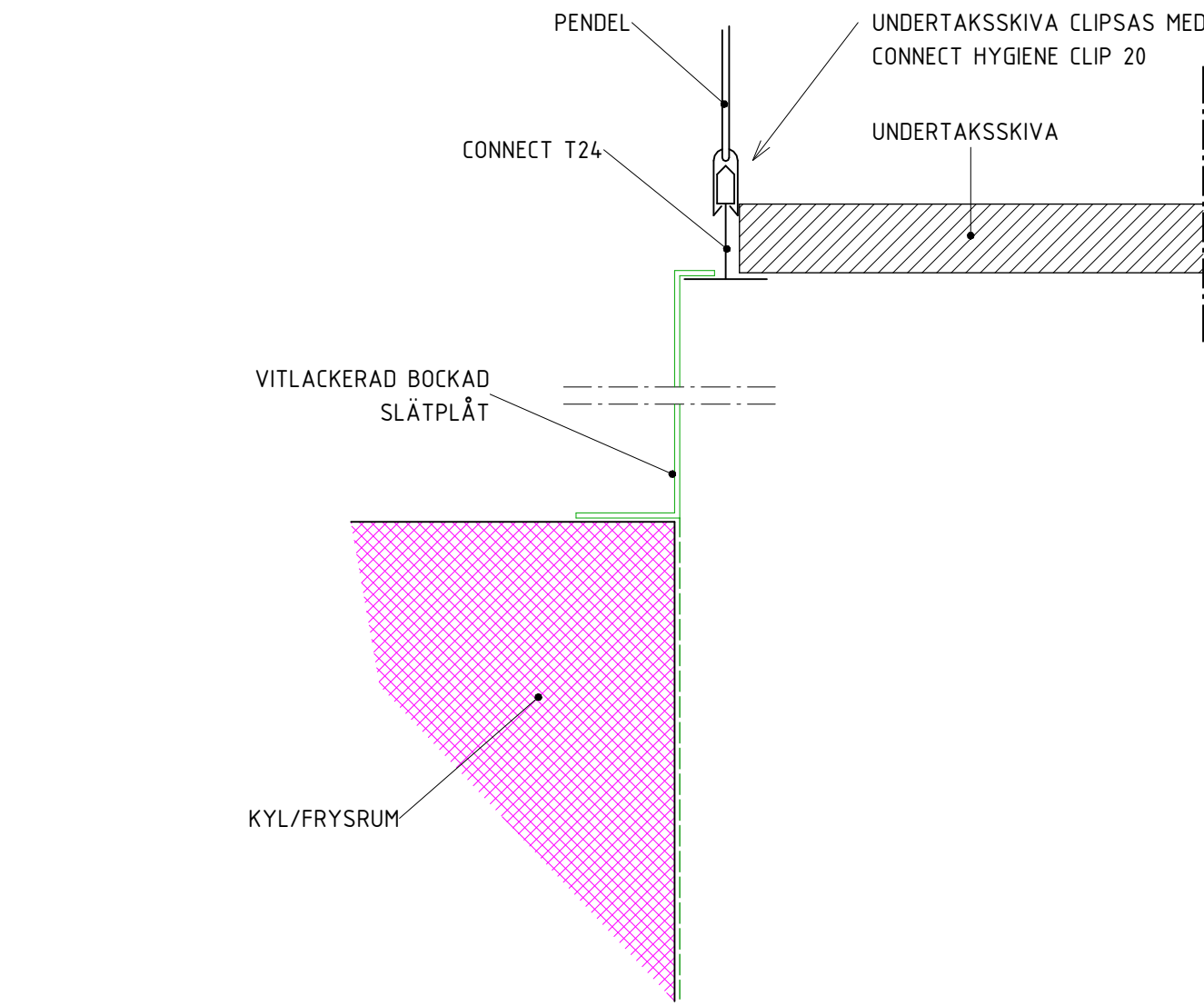
UTD02 - PRINCIPDETALJ ANSLUTNING MOT KYL-/FRYSRUM 1 : 2
