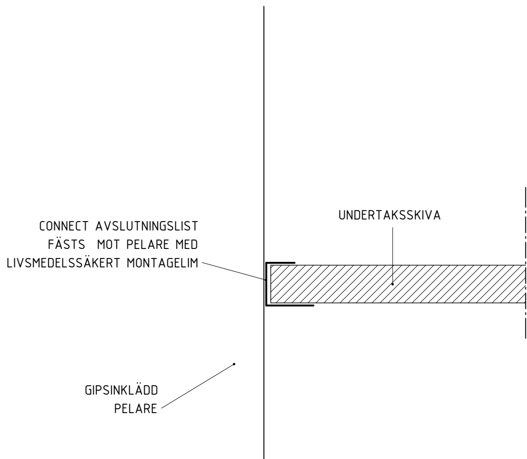
UTD06 - ANSLUTNING MOT PELARE 1 : 2
