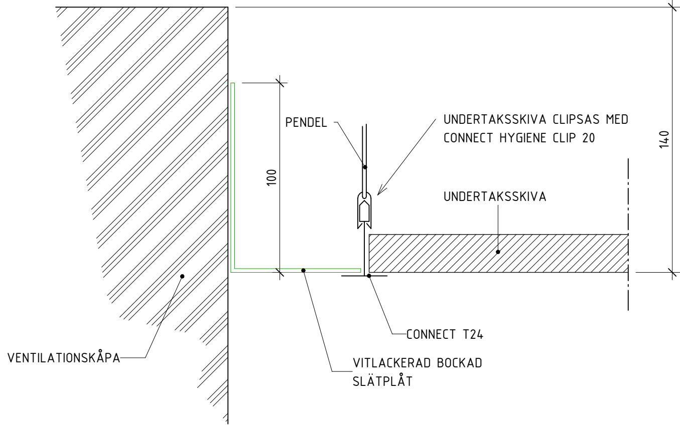
UTD04 - ANSLUTNING MOT VENTKÅPA 1 : 2
